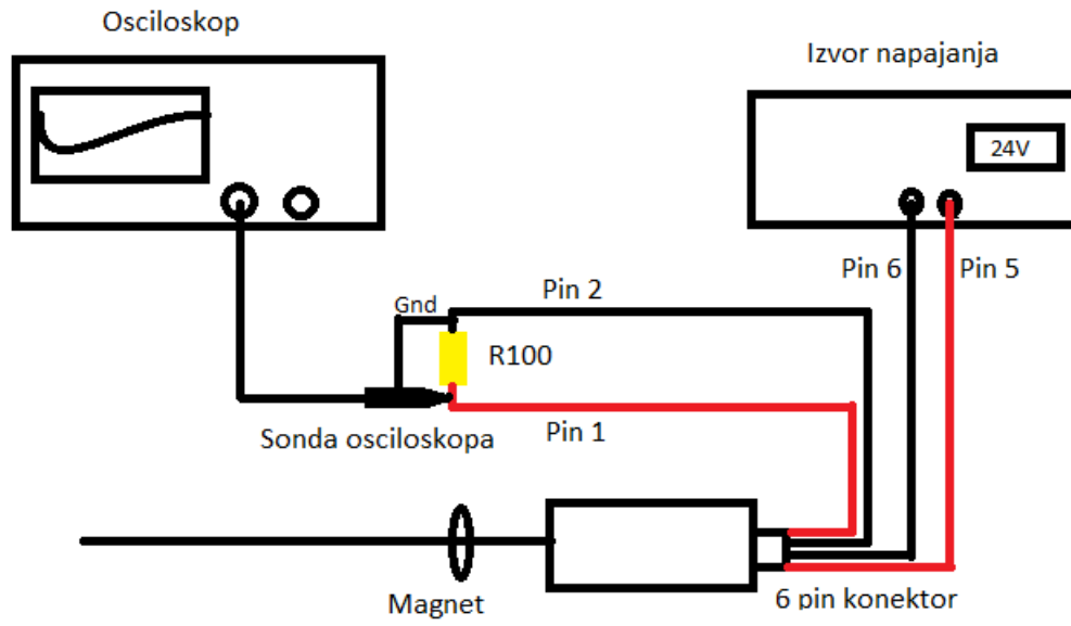
Slika 4.3. Shema mjernog spoja za snimanje dinamičke karakteristike.
