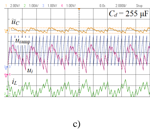
Slika 5.29 Utjecaj kapaciteta trošila na ustaljena stanja pretvarača; a) Simulacijom dobiveni bifurkacijski dijagrami s kapacitetima C_d = 165 \mu\text{F} i C_d = 255 \mu\text{F} , b) Valni oblici za E = 9,9 \text{ V} i C_d = 165 \mu\text{F} , c) Valni oblici za E = 9,9 \text{ V} i C_d = 255 \mu\text{F} .
