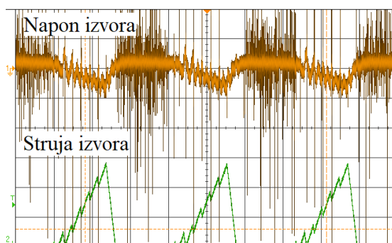
Slika 3.6 Propad napona izvora uzlaznog pretvarača pri najvećim opterećenjima. Osjetljivost je 50 \text{ mV/ds} i 2 \text{ A/ds} .
