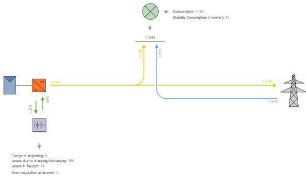
Slika 6.7 Tok energije [6]
