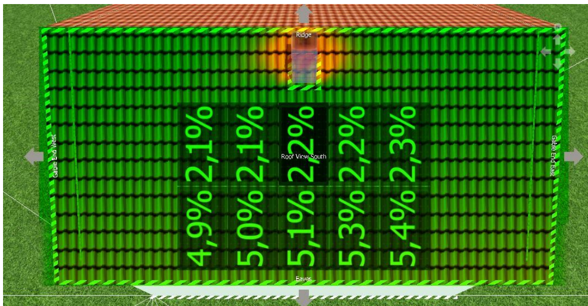
Slika 6.5 Zasjenjenje panela [6]
