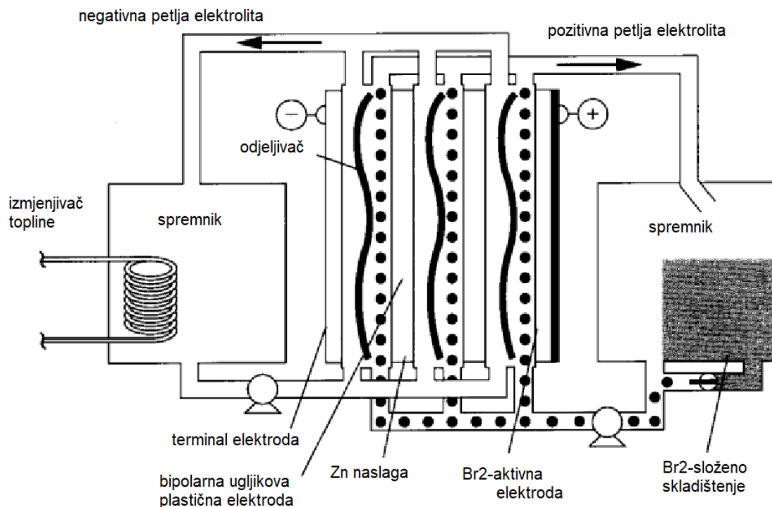
Slika 3.12 Struktura cink-bromidne baterije [1]
