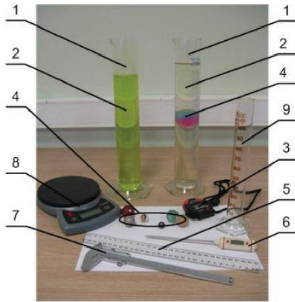
Slika 3.4. Pribor za izvođenje eksperimenta
