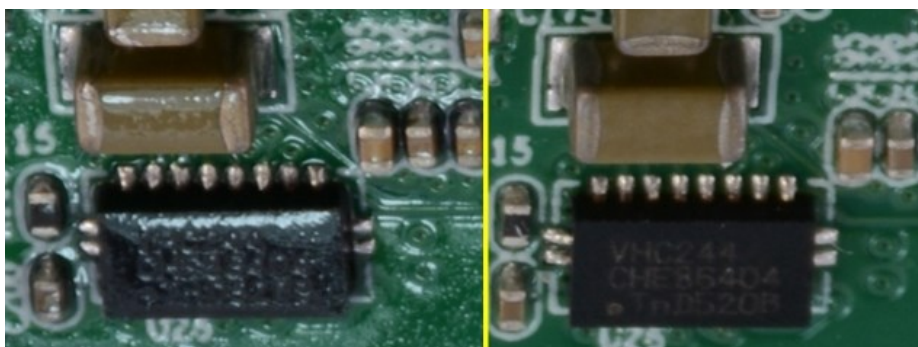
Sl. 4.1.4. Prikaz zaštite komponente komformnim premazom (lijevo) i bez zaštite (desno) [11]
