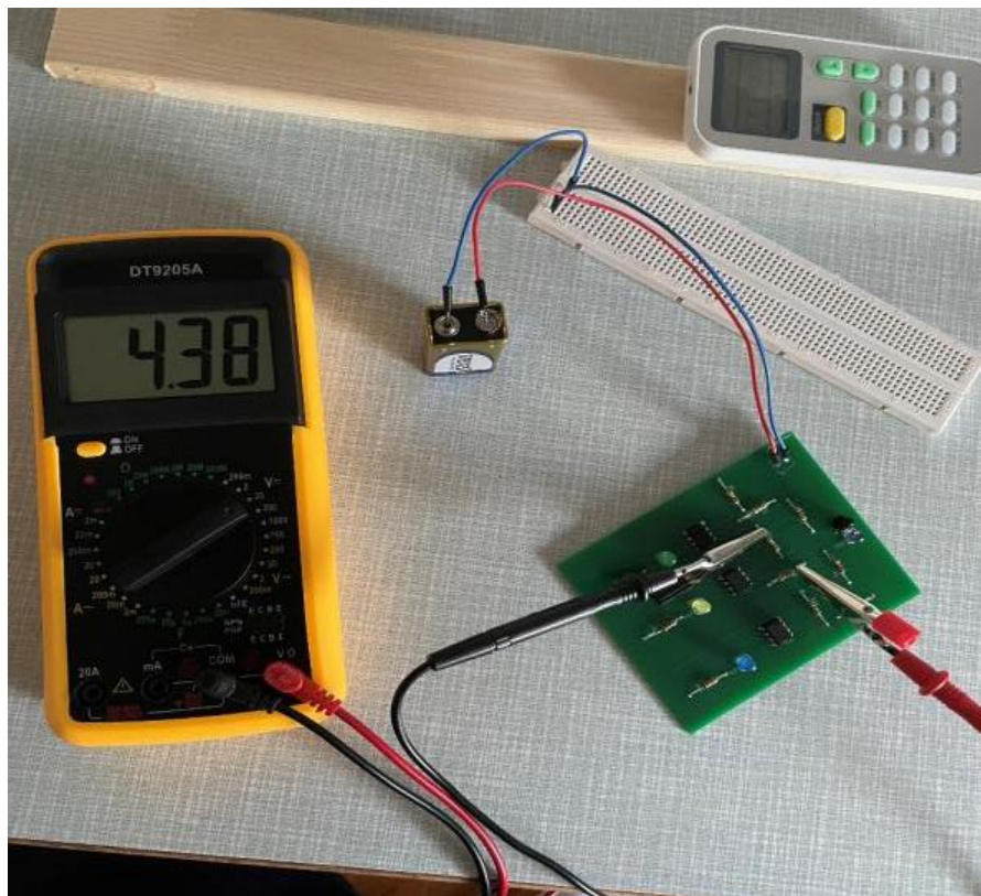
Slika 4.2. Rezultat mjerenja referentnog napona na otpornicima R4 i R8
