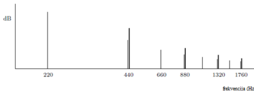
Slika 4.1 Osnovne frekvencije i njihove alikvote
