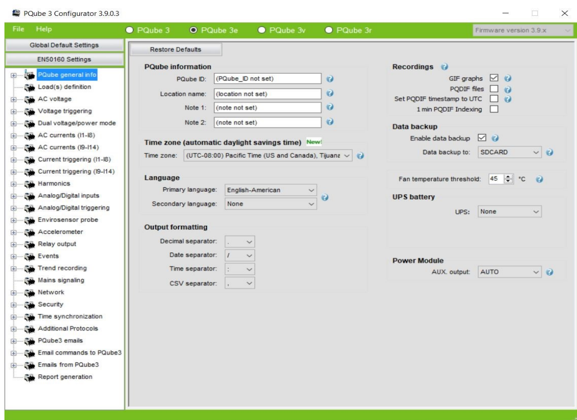
Slika 5.4 PQube 3 konfigurator
