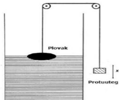
Slika 2.2. Prikaz mjernila s plovkom i formula za izračun parametara plovka [6]
