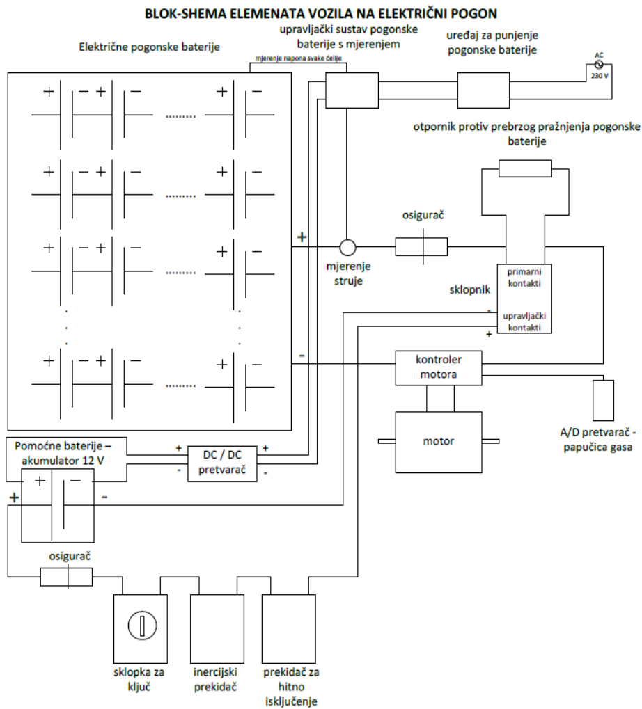
Slika 4.5 Blok struktura komponenti električnog vozila[25]
