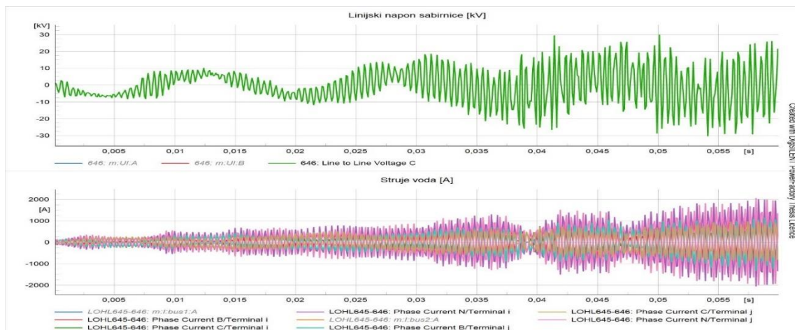
Slika 6.68 Prikaz valnog oblika linijskog napona na sabirnici 646 i struja na ulazu i izlazu voda LOHL645-646 poslije integracije punionica
