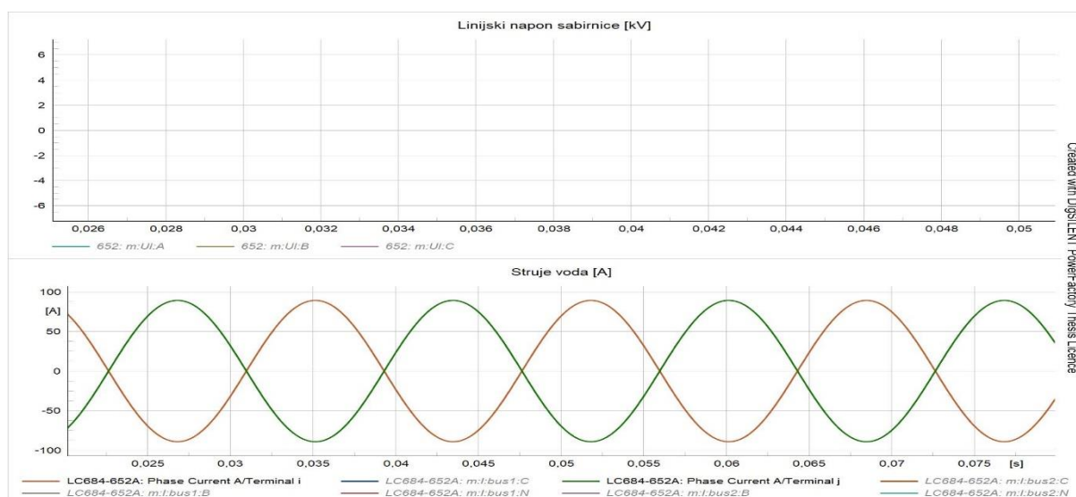
Slika 6.36 Prikaz valnog oblika linijskog napona na sabirnici 652 i struja na ulazu i izlazu voda LC684-652A prije integracije OIE
