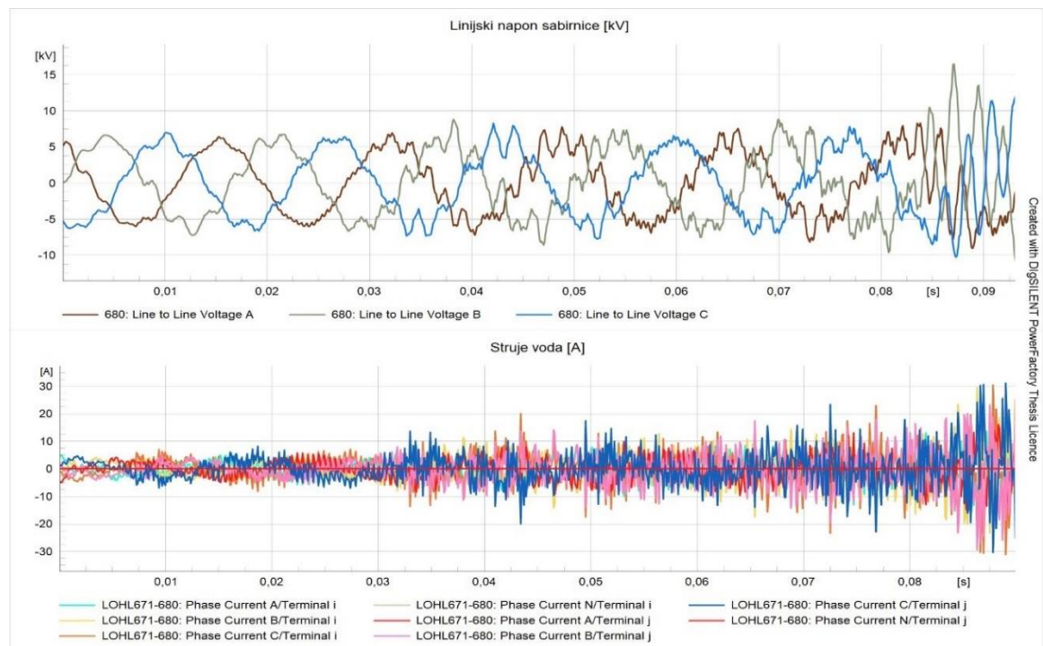
Slika 6.72 Prikaz valnog oblika linijskog napona na sabirnici 680 i struja na ulazu i izlazu voda LOHL671-680 poslije integracije punionica
