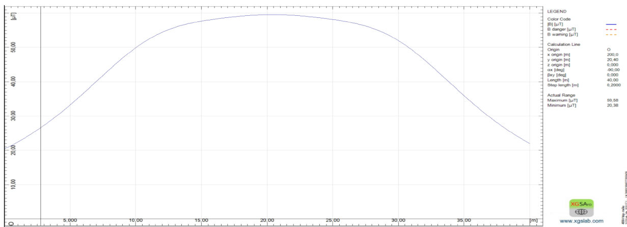
Slika 6.30. Magnetsko polje na površini zemlje (0 m)
