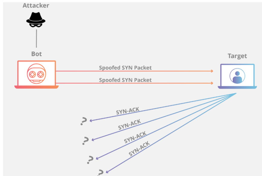
Slika 5.19: SYN flood [16]
