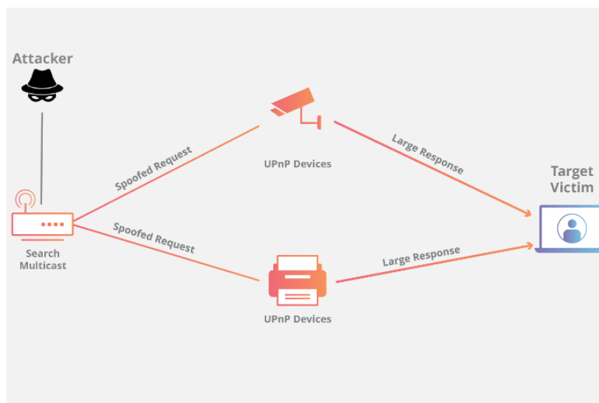
Slika 5.16: SSDP napad [16]
