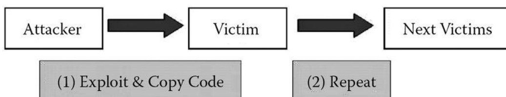
Slika 5.5: Autonomna propagacija [12]
