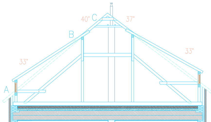
Slika 16: Presjek krovišta
