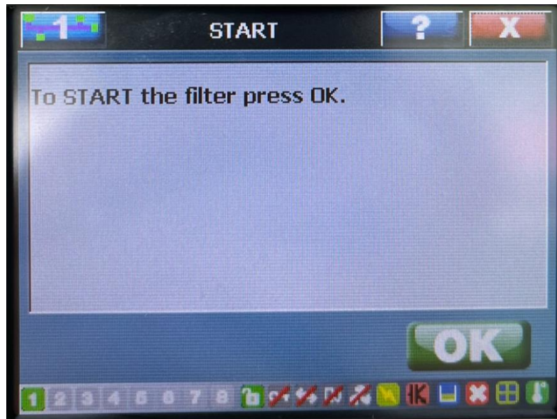
Slika 4.5. Pokretanje filtera
