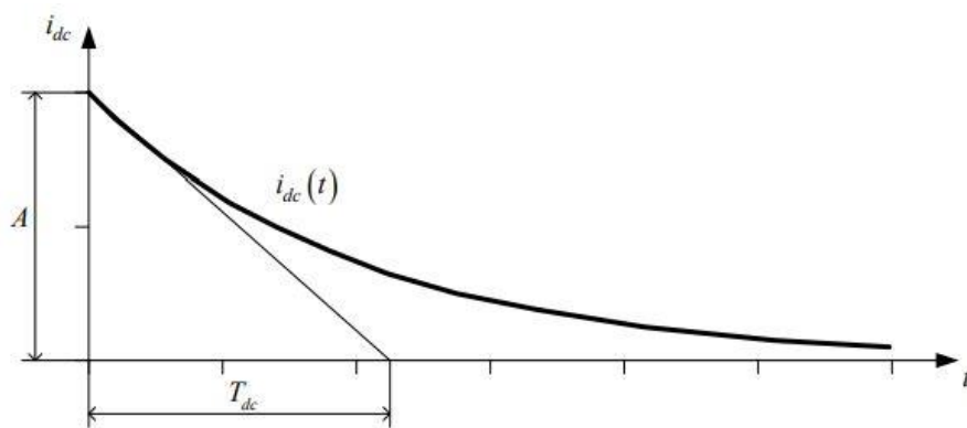
Sl. 5.2. Istopmjerna komponenta i_{dc}(t) [13]
