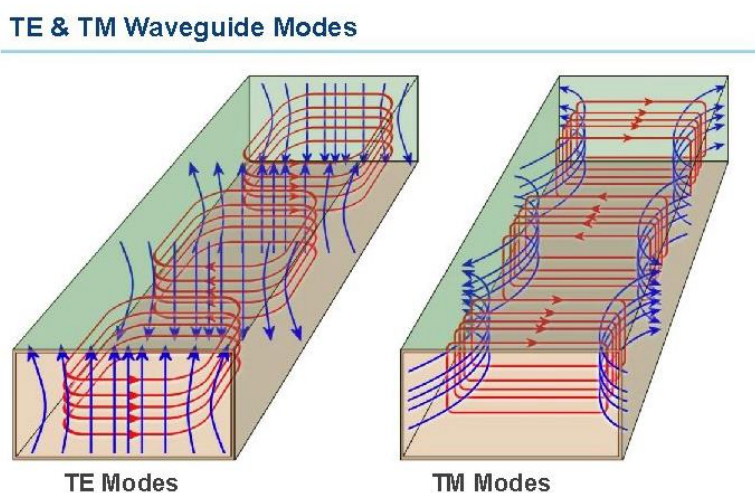
Slika 3.3. Različiti načini propagacije elektromagnetnog vala [11.]
