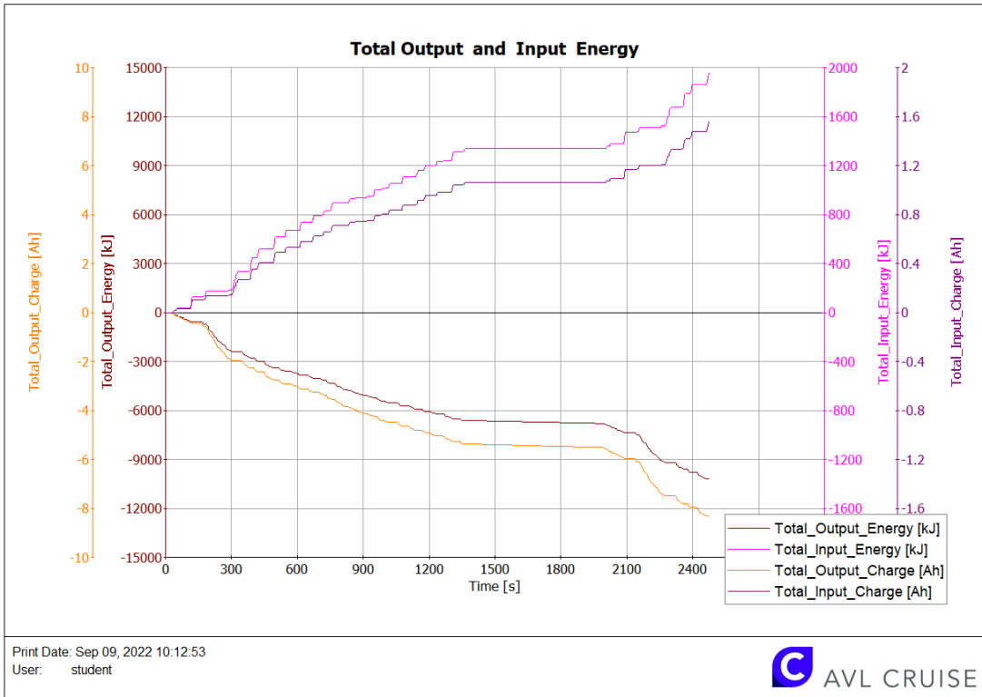
Slika 6.7. Dijagram ukupne izlazne i ulazne energije (FTP-75)
