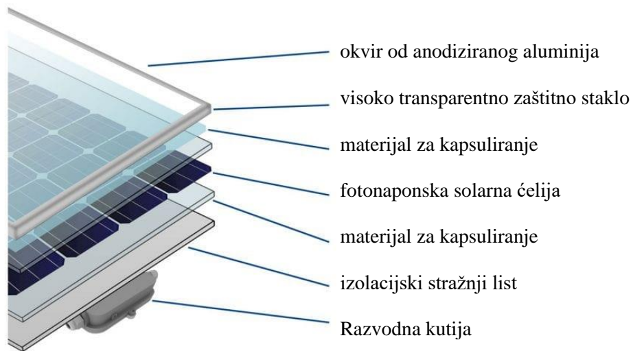
Slika 3.11, Prikaz sastava fotonaponske ćelije [24]
