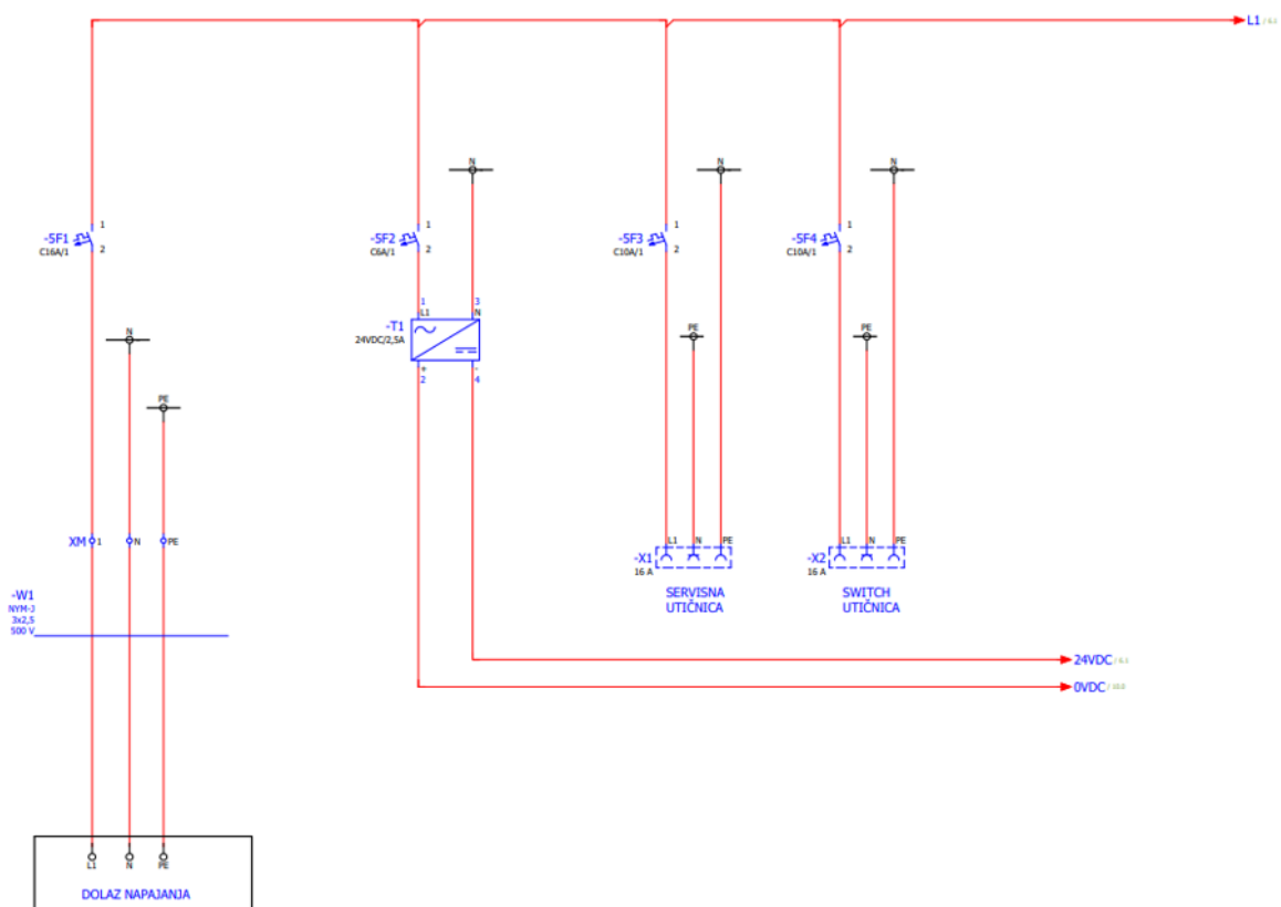
Slika 3.3 Dolazno napajanje
