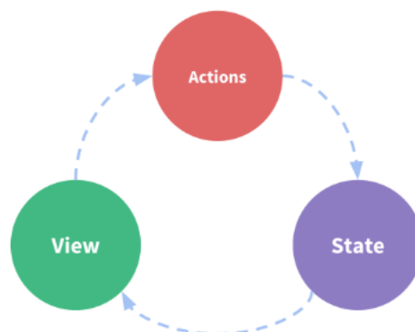
Slika 3.9. Prikaz zajedničkog rada dijelova Vuex store-a
