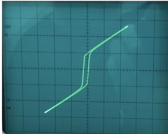
Slika 5.11. Petlja histereze CRGO uzorka
