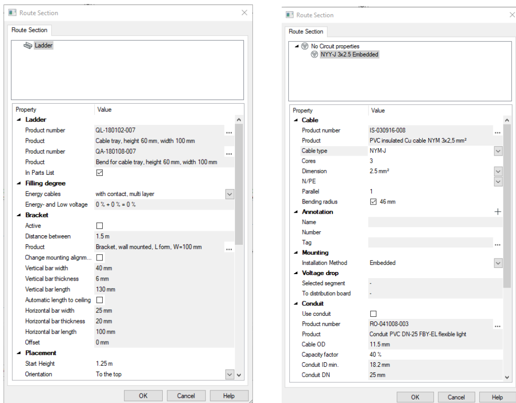
Slika 4.12 Definiranje kabelskih polica (lijevo) i kabela (desno)
