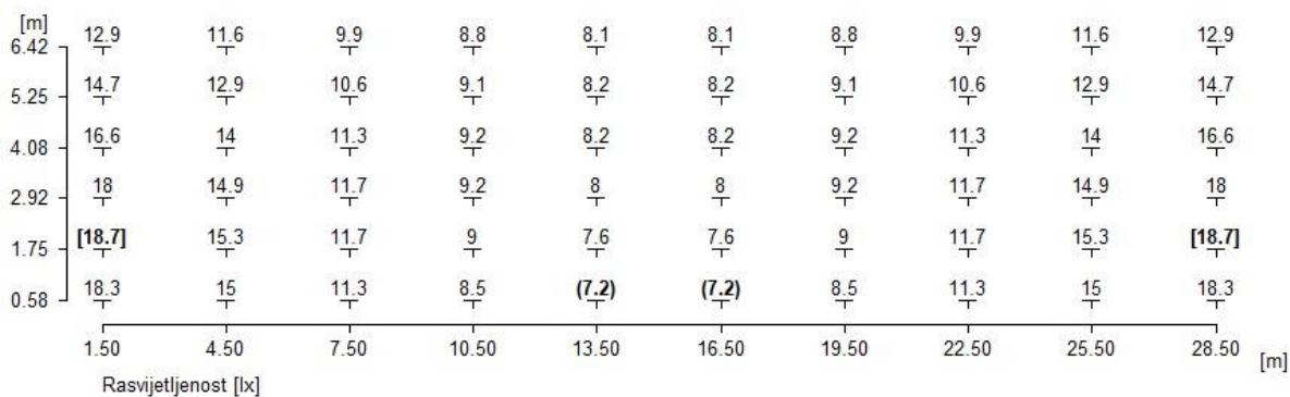
Sl. 4.8. Vrijednosti rasvjetljenosti odabrane svjetiljke
