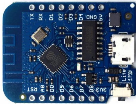
Sl. 3.3. Wemos D1 mini Lite
