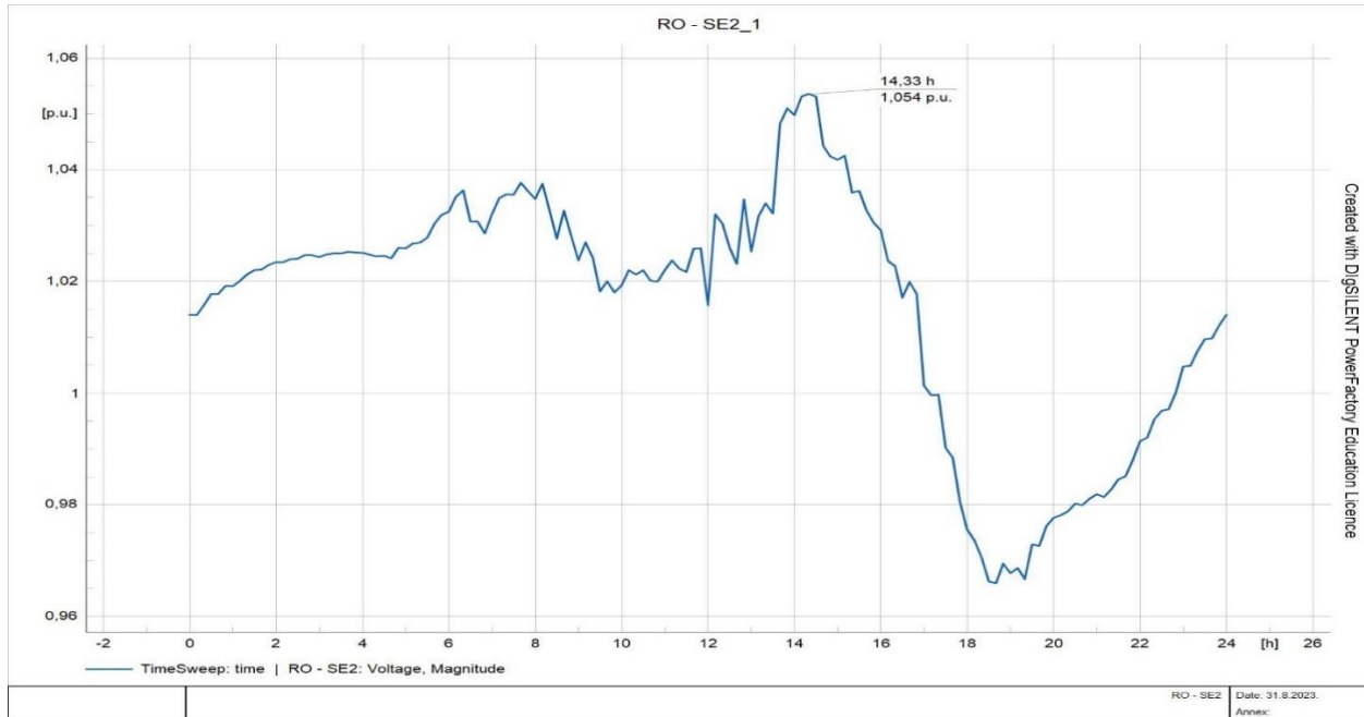
4.39. Dijagram napona na sabirnici RO-SE2 nakon promjene \cos\phi na 0,9 ind.
