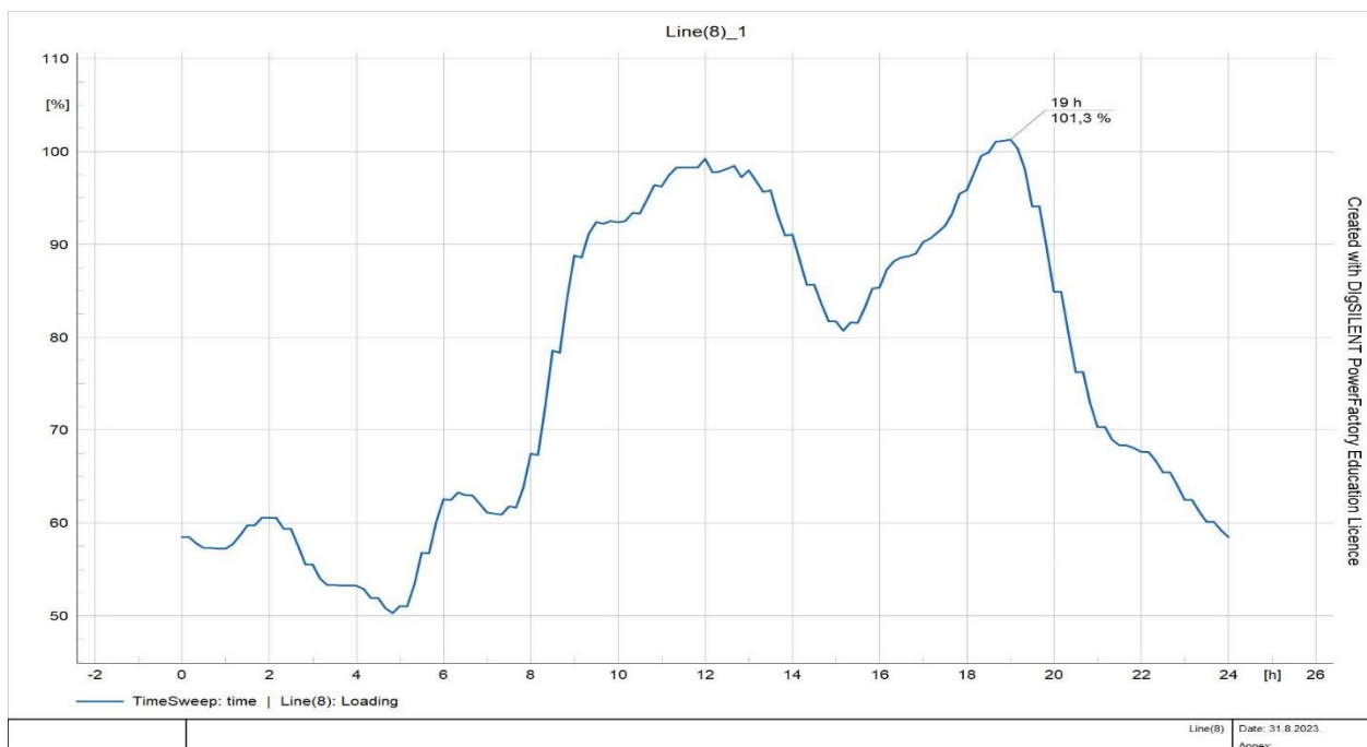
4.40. Opterećenje voda do sabirnice INA nakon promjene \cos\phi na 0,9 ind.
