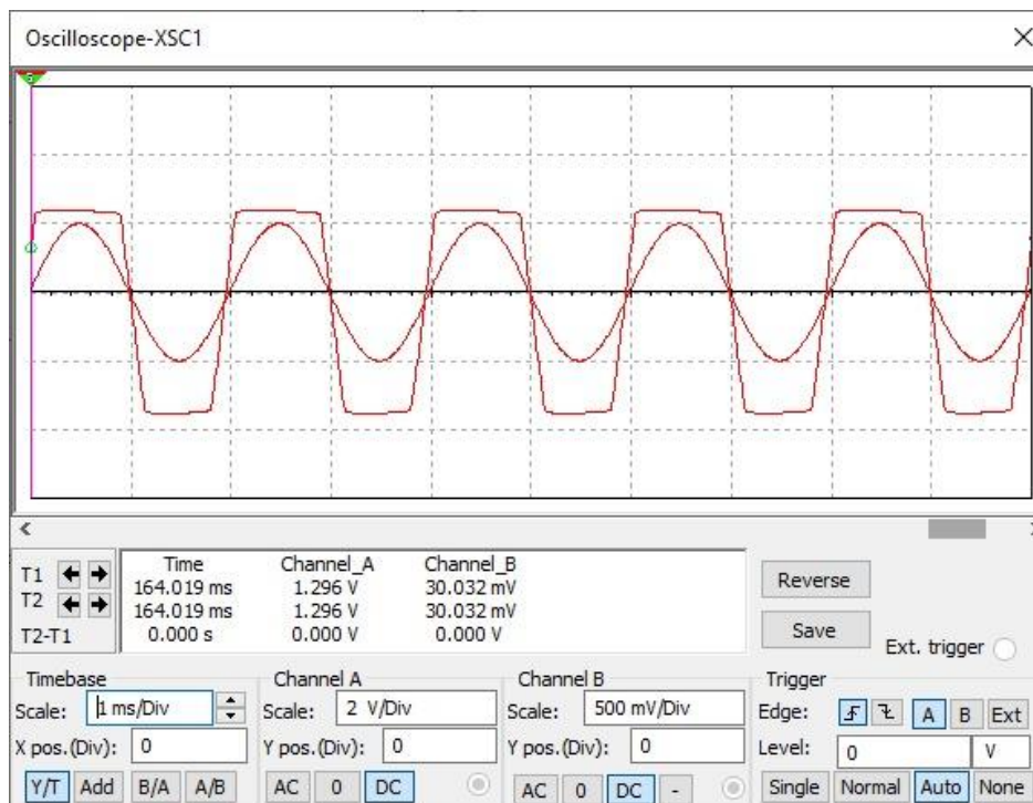
Slika 6.9: Prikaz ulaznog i izlaznog signala kada je potencijometar L i C postavljen na 0% pri amplitudi 600 mVpp i frekvenciji 500 Hz
