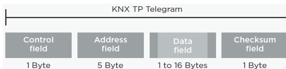
Slika 3.2. KNX TP telegram
