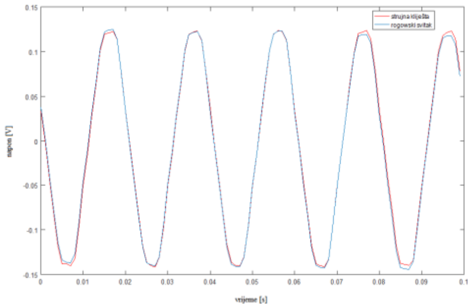
Slika 5.4. Signal sinusnog oblika izmjeren sa Rogowskijevim svitkom i strujnim klijestima u slučaju kada je mjerni vodič u središtu Rogowskijevog svitka. [24]
