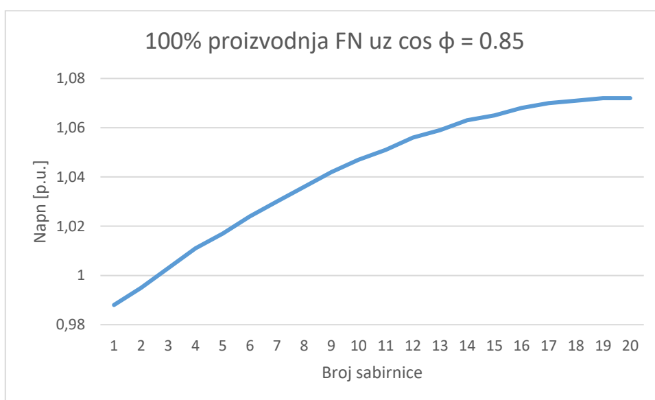
Slika 4.70. Napon na sabirnicama pri \cos \varphi = 0,85 (maksimalna proizvodnja FN-a)
