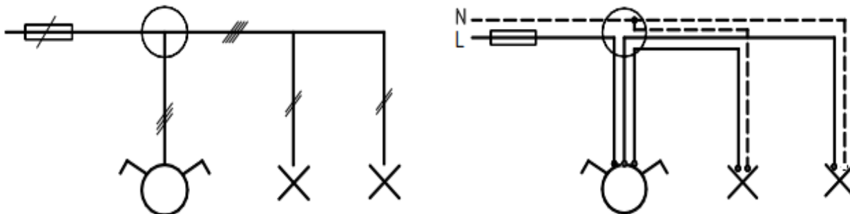
Slika 2.3. Primjer sheme strujnog kruga s dva rasvjetna mjesta (serijska sklopka), jednopolna i višepolna shema. [1]
