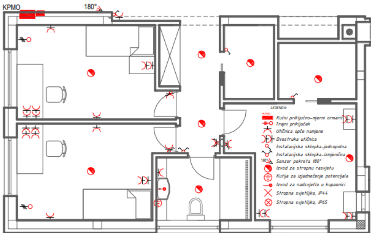
Slika 2.5. Primjer sheme električne instalacije u kući. [1]
