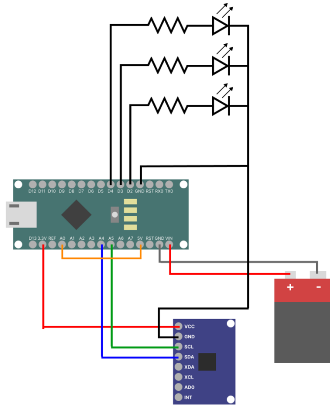
Slika 3.5. Nacrt potpunog spoja
