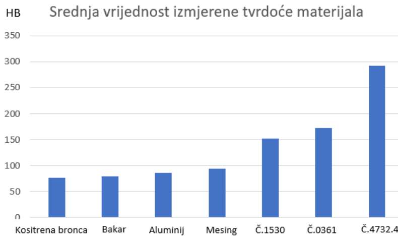
Sl.4.3.Graf srednjih vrijednosti izmjerene tvrdoće materijala stacionarnim tvrdomjerom
