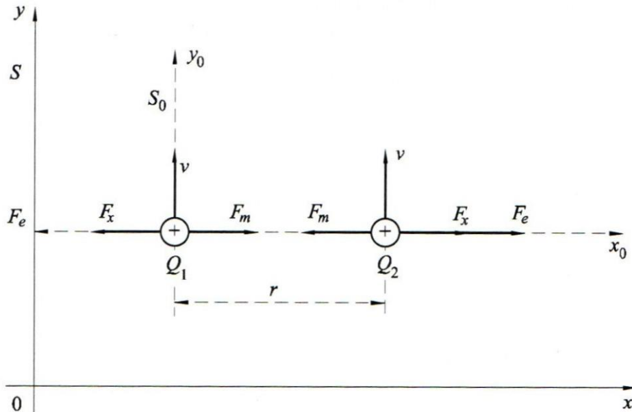
Slika 4.4. Sila između dvaju mirnih naboja u inercijalnom sustavu S_0 koji se giba brzinom v u odnosu na mirni inercijalni sustav S [1]
