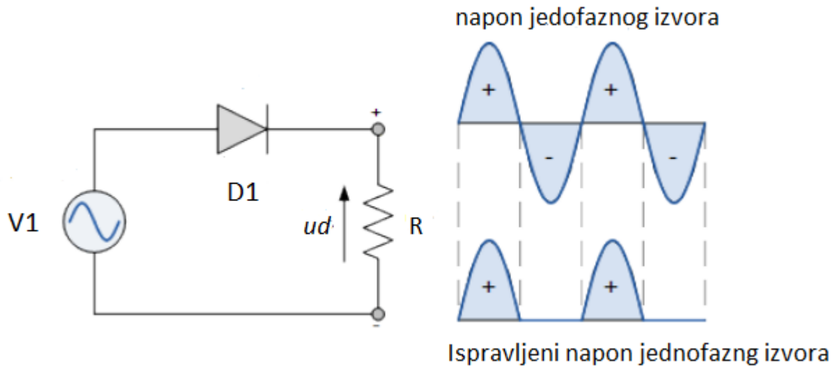
Slika 4.10. Ispravljanje napona diodom [21]
