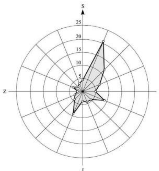
Slika 3.2 Ruža vjetrova [12]
