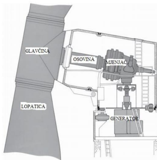
Slika 4.11 Generator u vjetroturbini [18]
