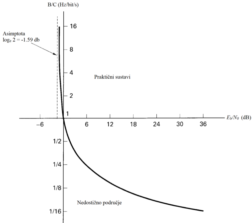
Slika 4.4. Normalizirana propusnost kanala u odnosu na kanal E_b/N_0
