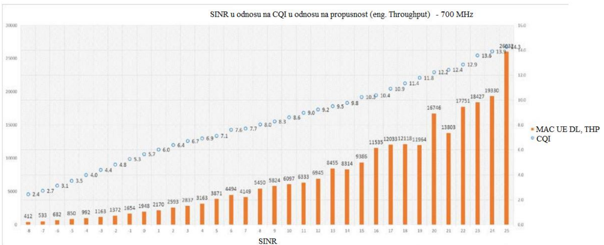
Slika 4.7. SINR - CQI - UE propusnost (Kbps) korelacija [22]
