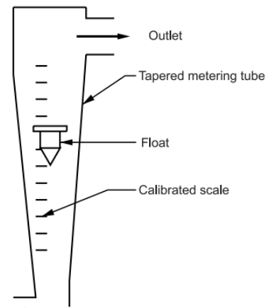
Slika 4.21 Načelo rada rotametra [21]
