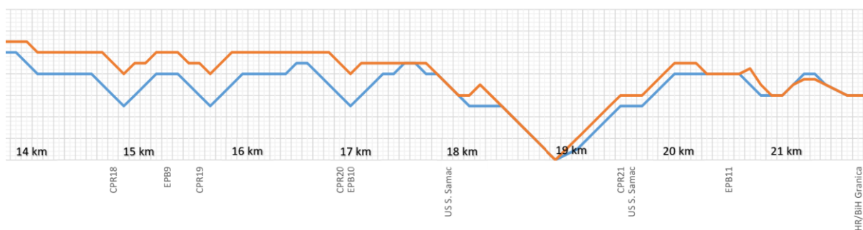
Slika 6.10. – Dijagram brzine vlaka od km 14 do km 22 na sekciji pruge: Vrpolje – Državna granica HR
