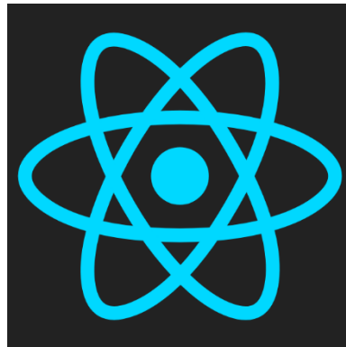
Slika 3.4. React logo.
