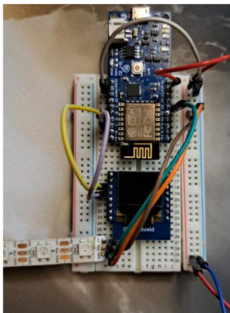
Sl. 3.17. Sklop u početnom stadiju izrade
