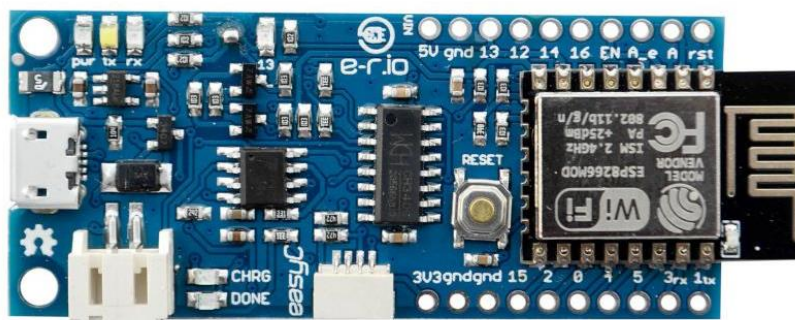
Sl. 3.1. Croduino Nova 2
