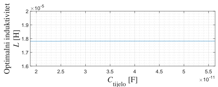
(a) Ovisnost optimalnog induktiviteta L o parametru C_{tijelo}
