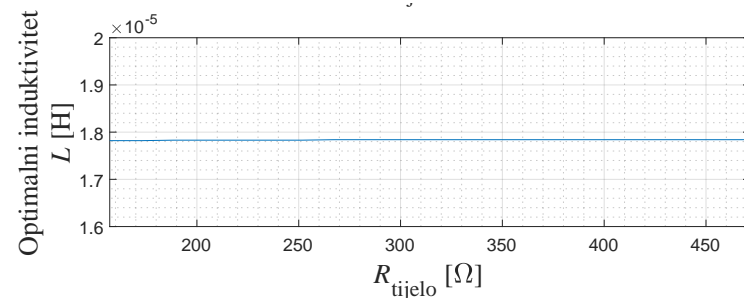
(b) Ovisnost optimalnog induktiviteta L o parametru R_{tijelo}
