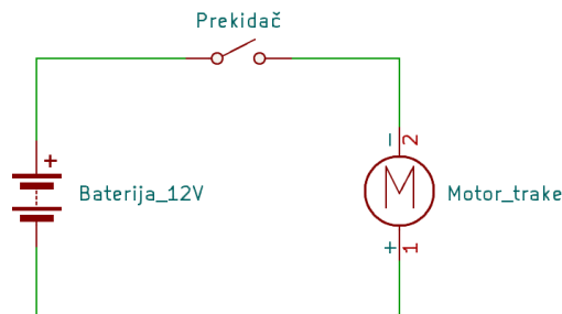
Slika 3.9. Električna shema spoja motora za pokretanje trake
