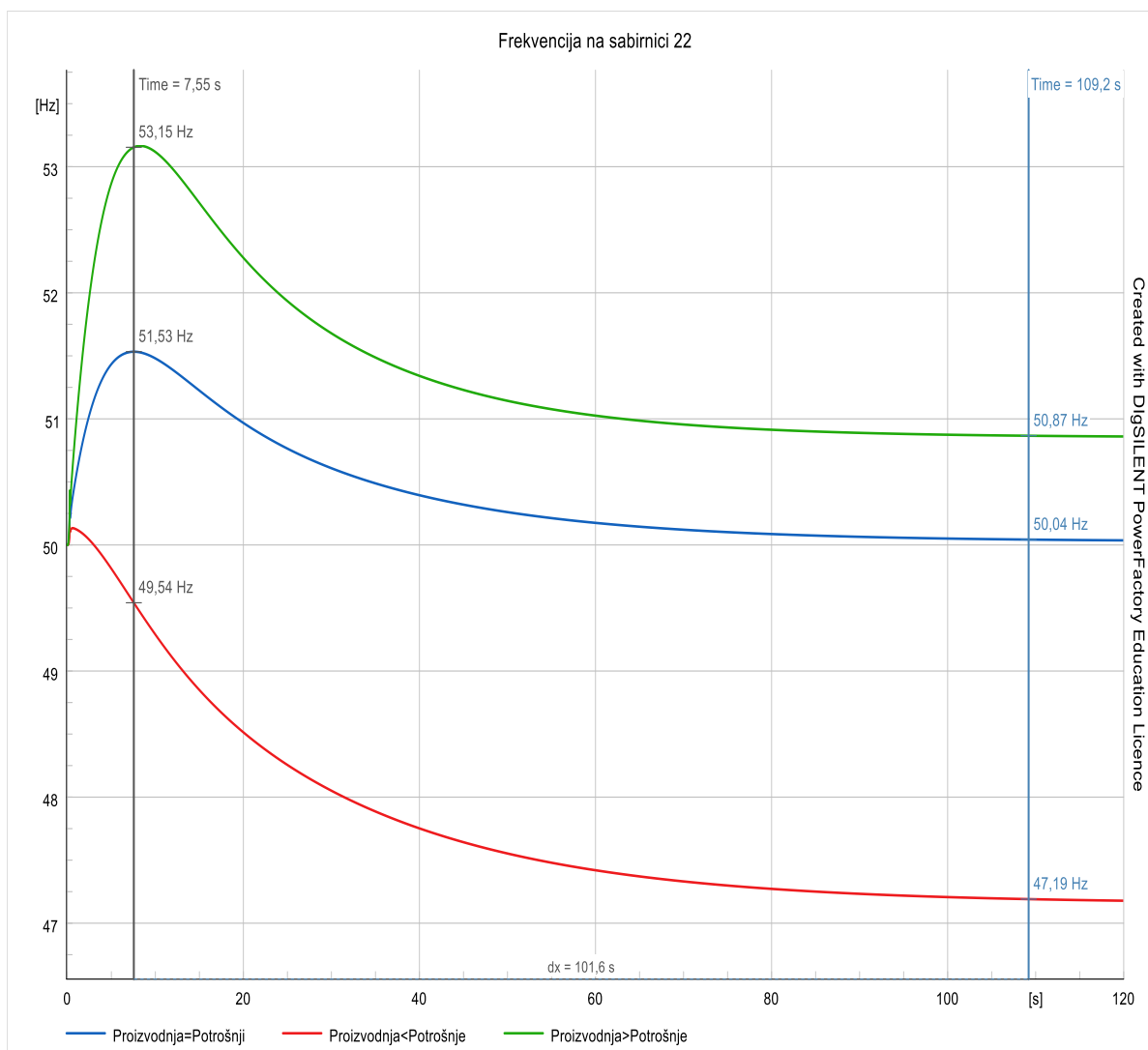
Slika 4.23. Sabirnica 22 – frekvencija – ustaljeno stanje
