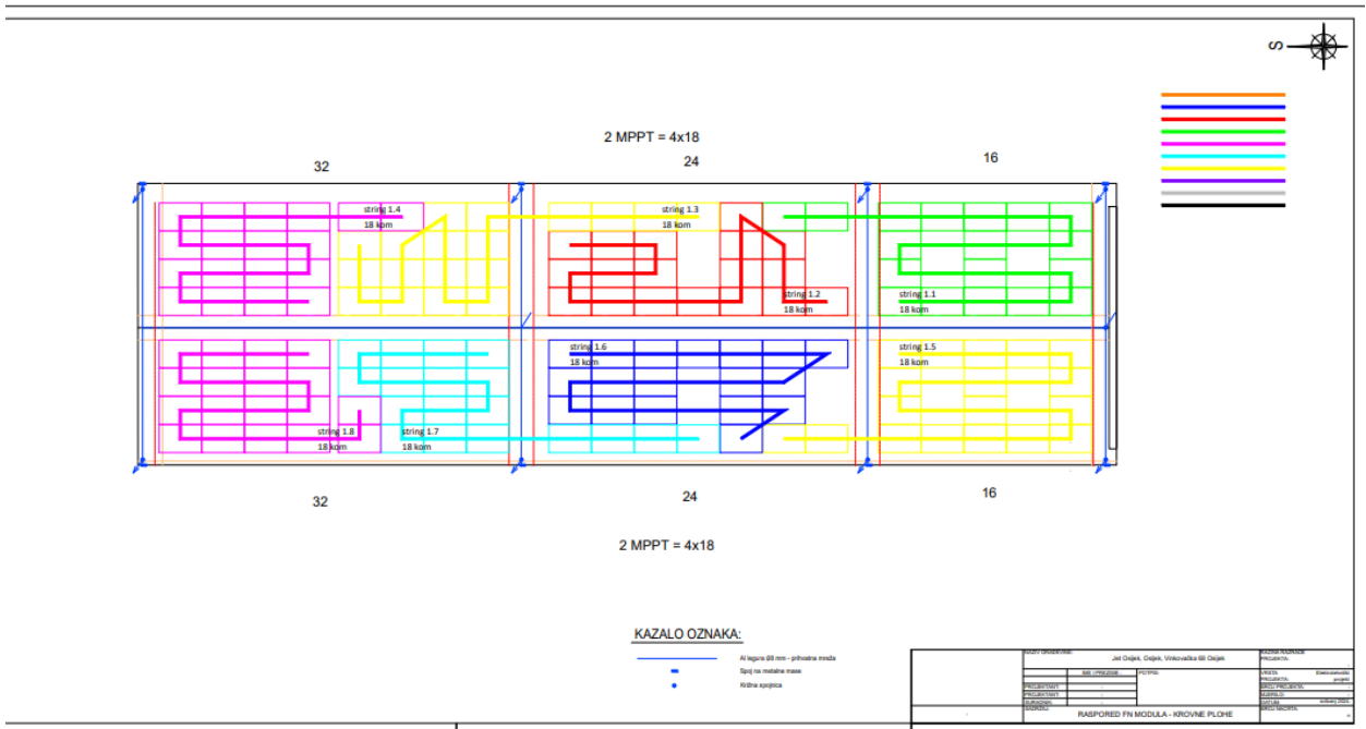
Slika 4.33. Rezultat rada u AutoCAD-u koji prikazuje tlocrt građevine sa ucrtanim FN modulima i gromobranima [15]
