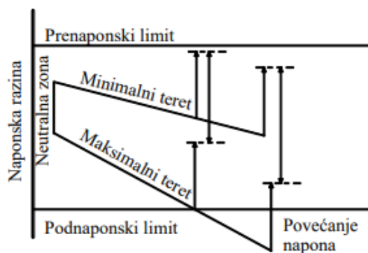
Slika 3.3. Usklađivanje napona duž distributivnog voda; Apscisa prikazuje udaljenost od glavne SN trafostanice na sekundarnoj strani VN/SN transformatora, dok ordinata prikazuje napon na sekundarnoj strani SN/NN transformatora na ovom mjestu [1]
