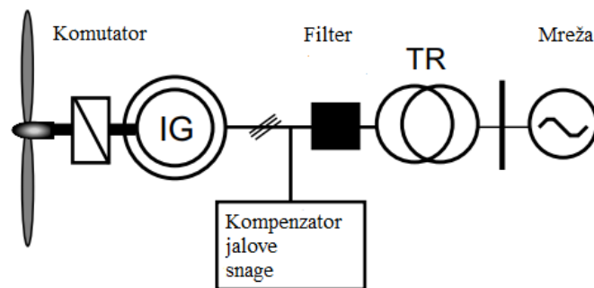
Slika 2.4. Izravni priključak vjetroturbine na mrežu preko asinkronog generatora i kompenzatora jalove snage [1]
