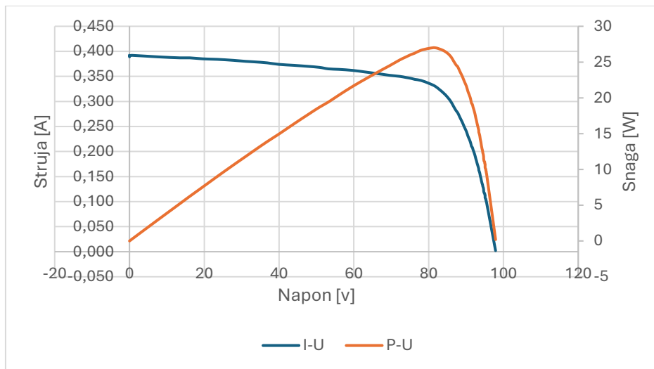
Slika 6.21. I-U i P-U karakteristike modula Solar Frontier SF-150 pri zasjenjenju prvog reda
