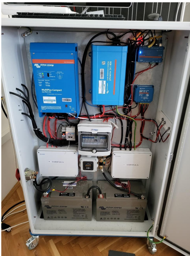
Sl. 5.1. Mikromreža
