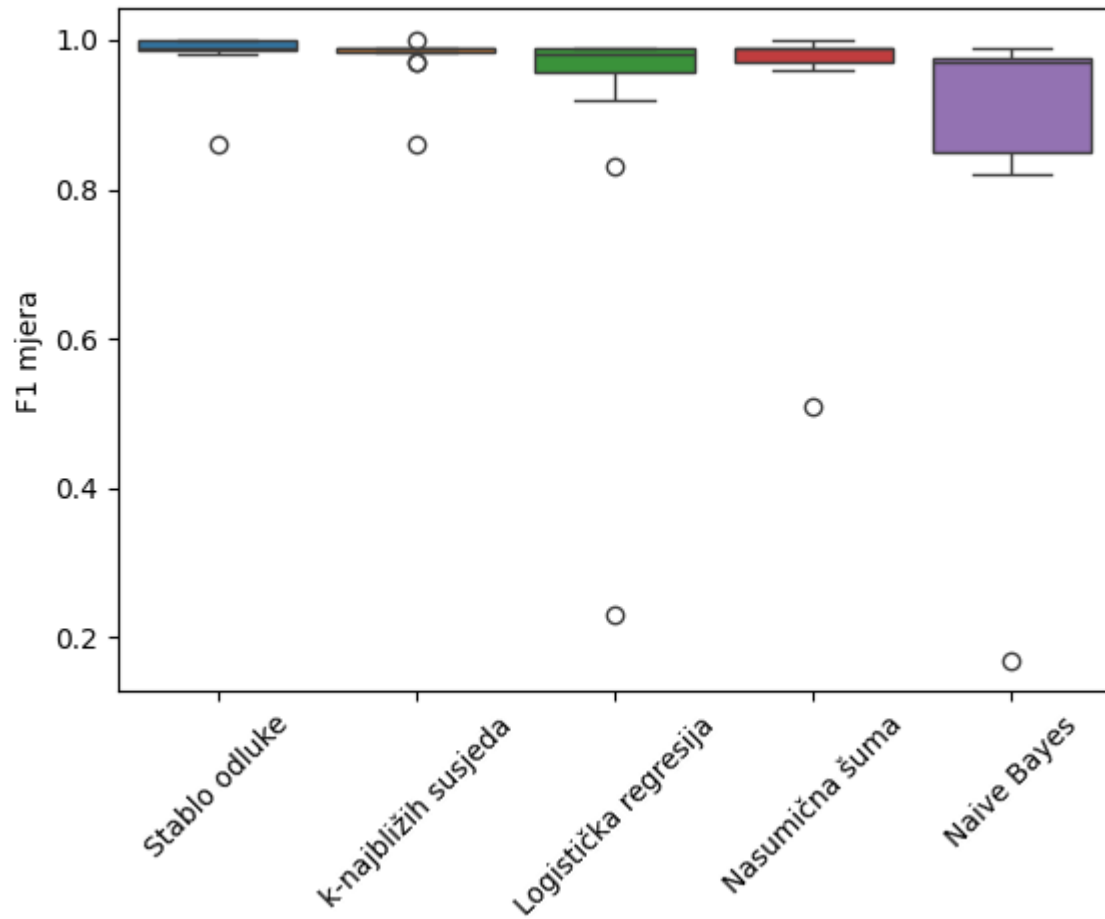
Sl. 4.1. Dijagram pravokutnika vrijednosti F1 mjera za svaki klasifikacijski algoritam
