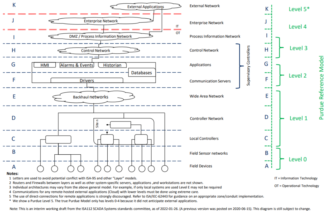
Slika 3.1. Dijagram arhitekture modela SCADA sustava [4]
